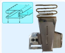
DOBLADILLADOR RECTO
