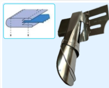
DOBLADILLADOR FONTRAL
