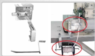
GUIADOR INFERIOR PARA ELÁSTICO (ART. 18316)
