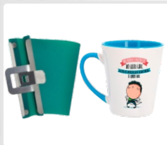
ABRAZADERA (TAZA / 12 ONZAS / CÓNICO) ART. 21306
