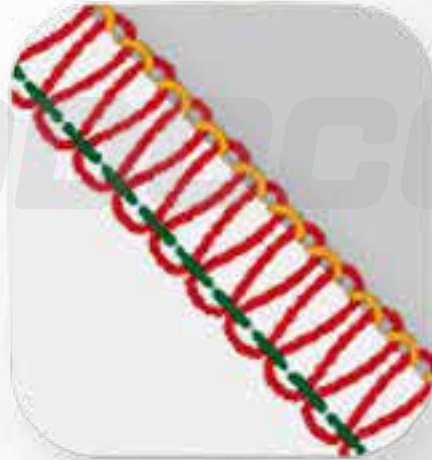
OVERLOCK ESTRECHO DE 3 HILOS
